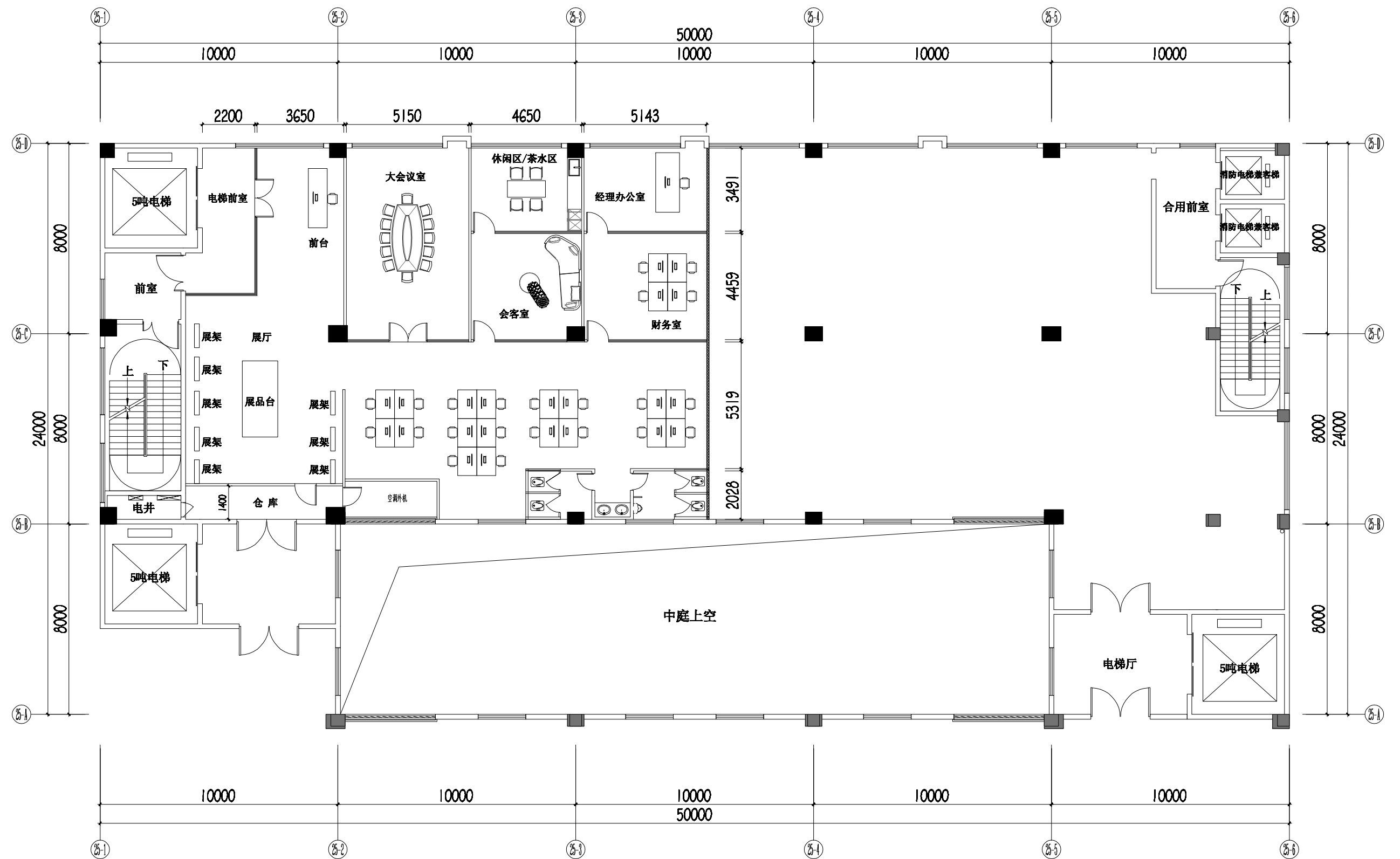
平面布置图
